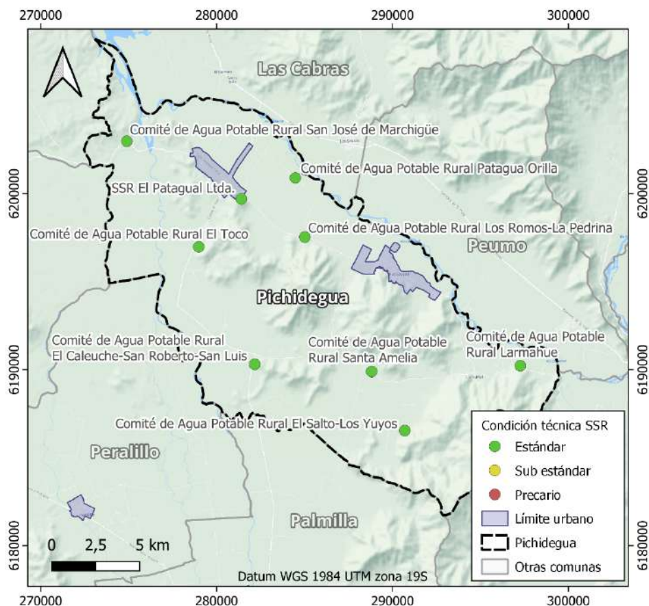
Figura 3-11. Ubicación de Servicios Sanitarios Rurales en operación y con resolución sanitaria vigente a junio de 2024 en la comuna de Pichidegua
